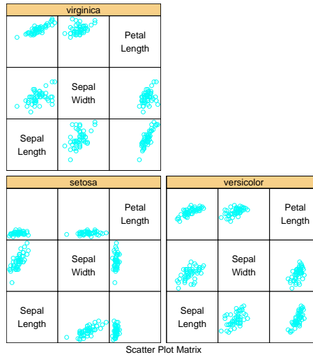
FIG. 11 – La fonction spIom avec les données « iris » (2).
