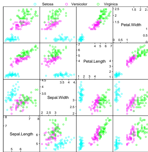
FIG. 10 – La fonction spIom avec les données « iris » (1).
